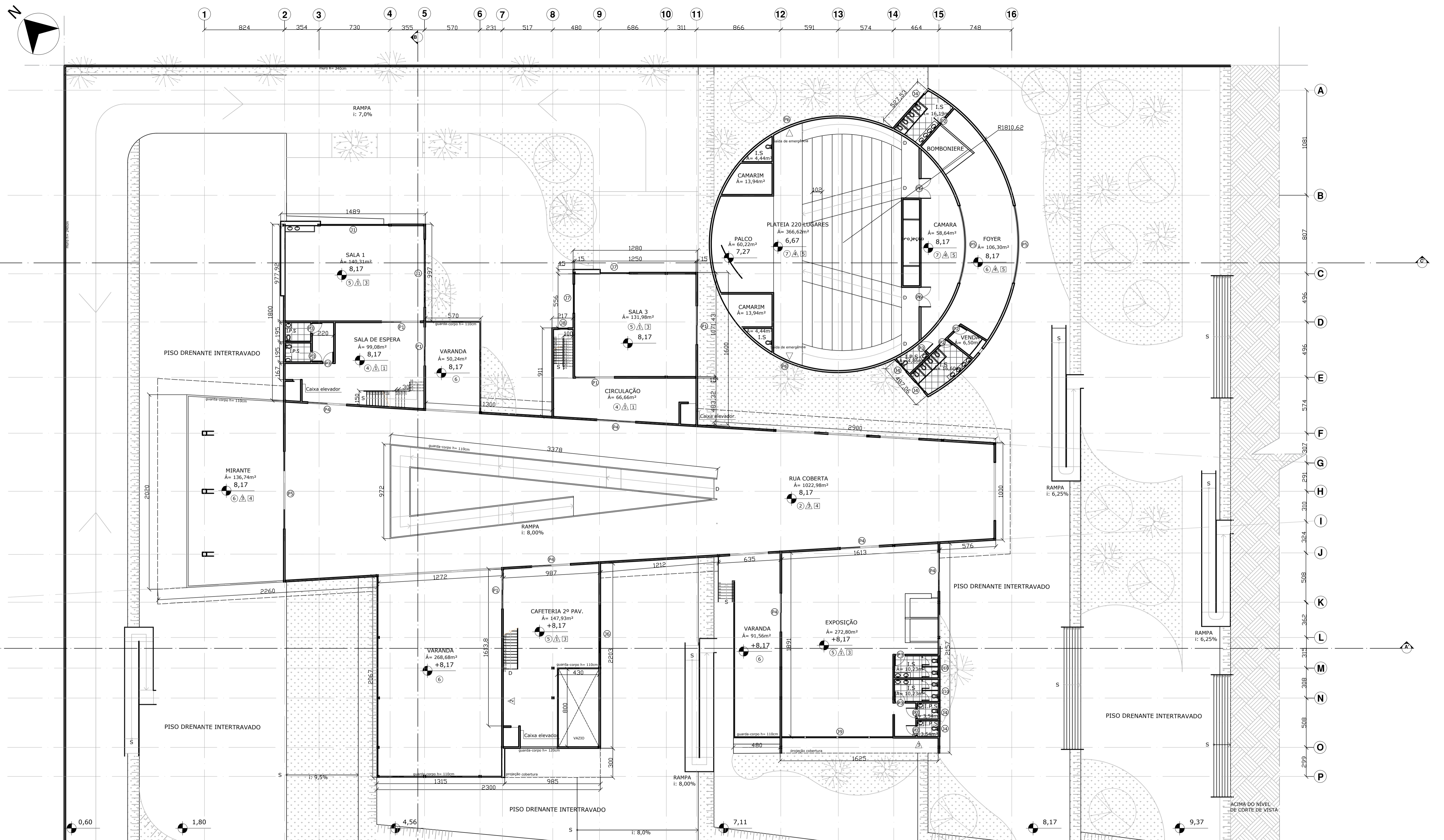
08 PLANTA NÍVEL 8,17 ESC. 1/200
