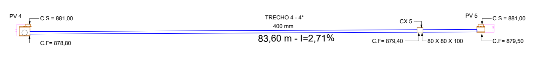
4 TRECHO 4 - 4* 1:600
