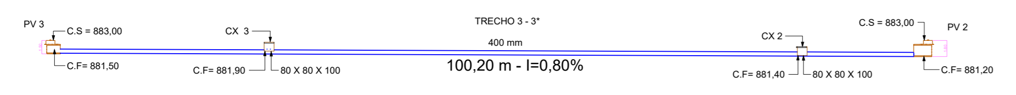
3 TRECHO 3 - 3* 1:600
