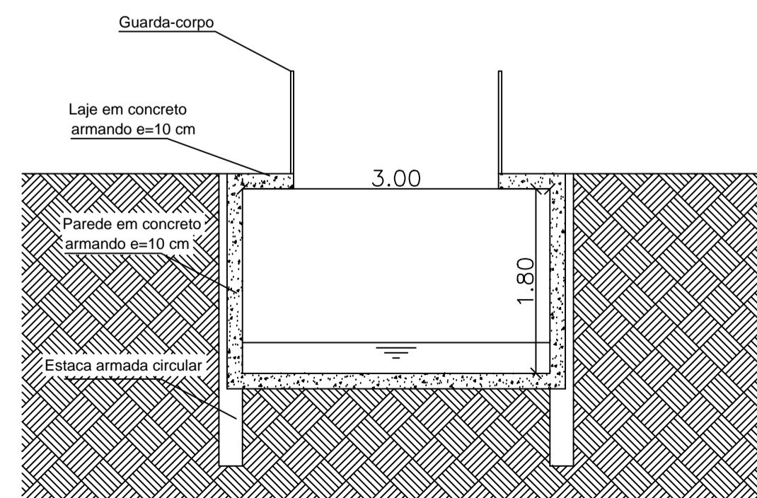
Trecho19 Escala 1:50
