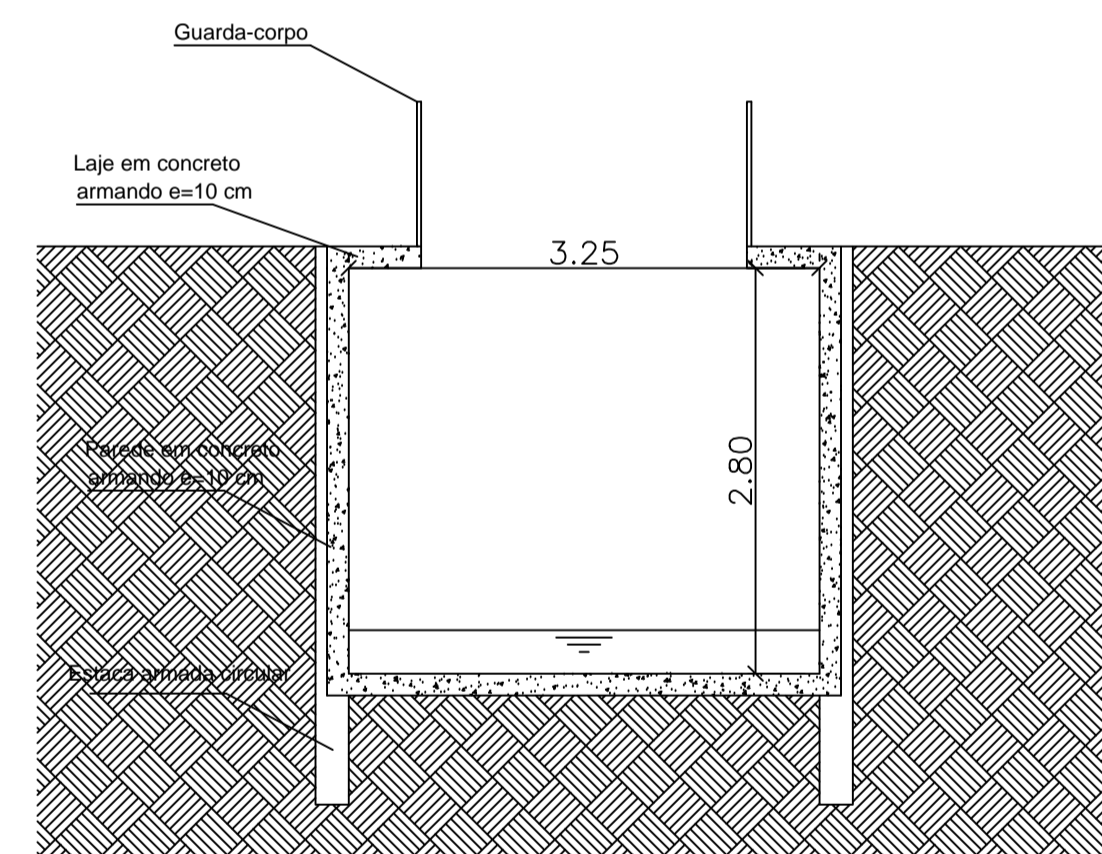
Trecho18 Escala 1:50
