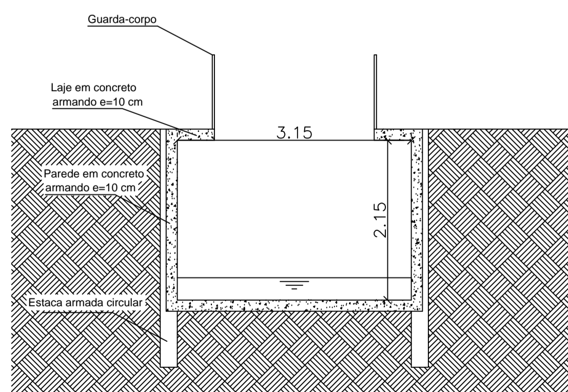
Trecho 9 Escala 1:50
