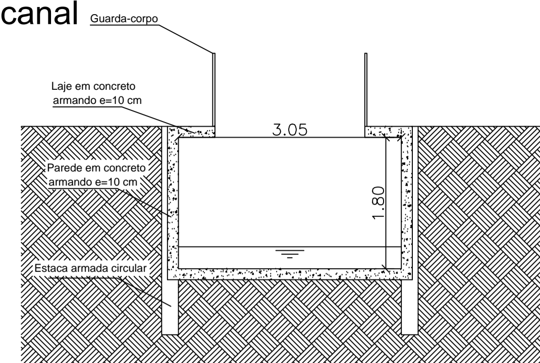
Trecho14 Escala 1:50
