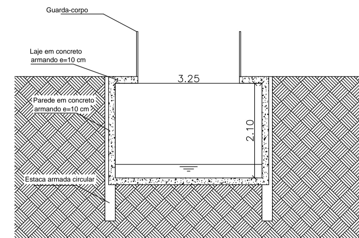
Trecho 8 Escala 1:50
