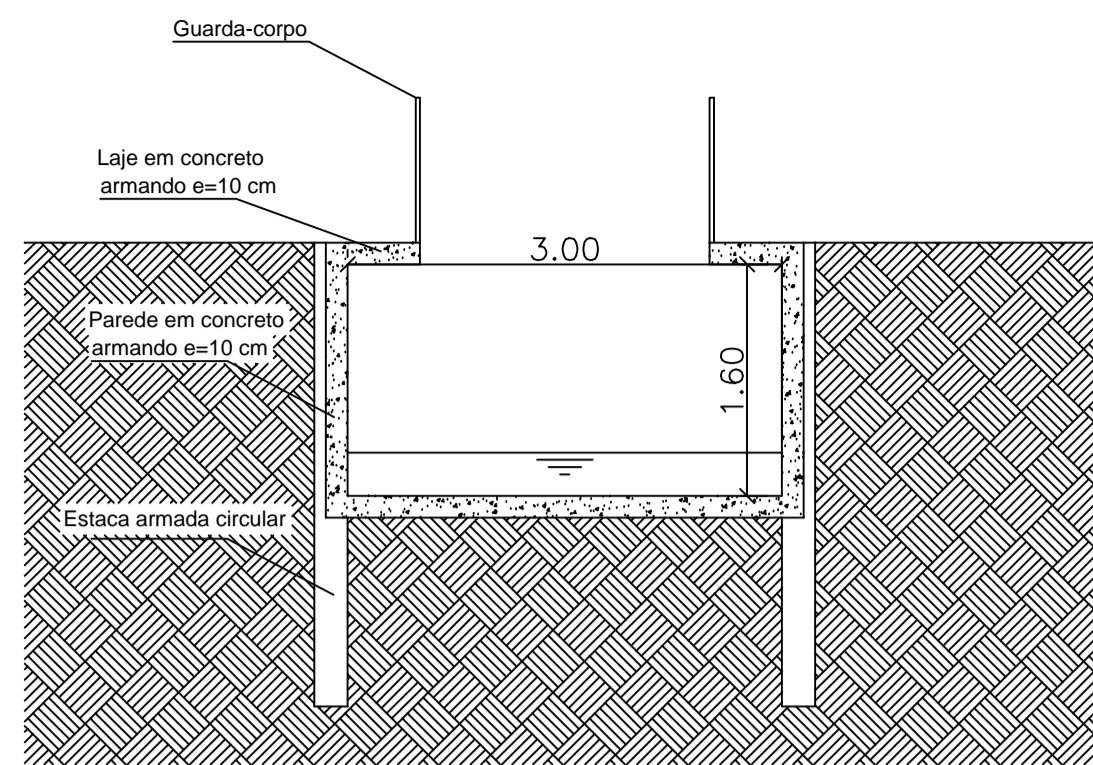
Trecho 6 Escala 1:50
