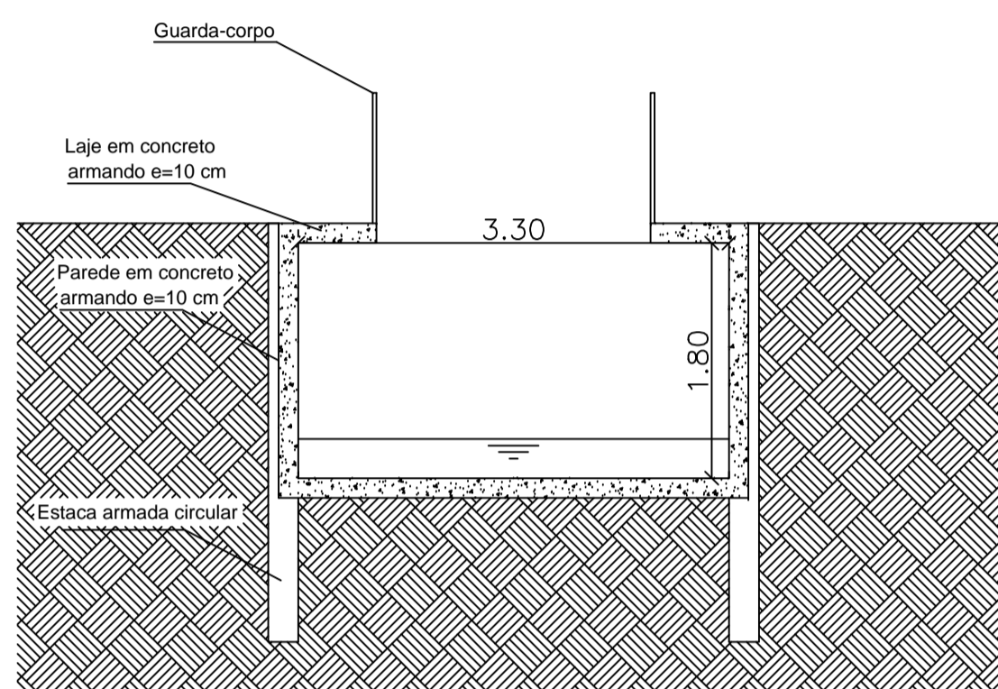
Trecho 7 Escala 1:50
