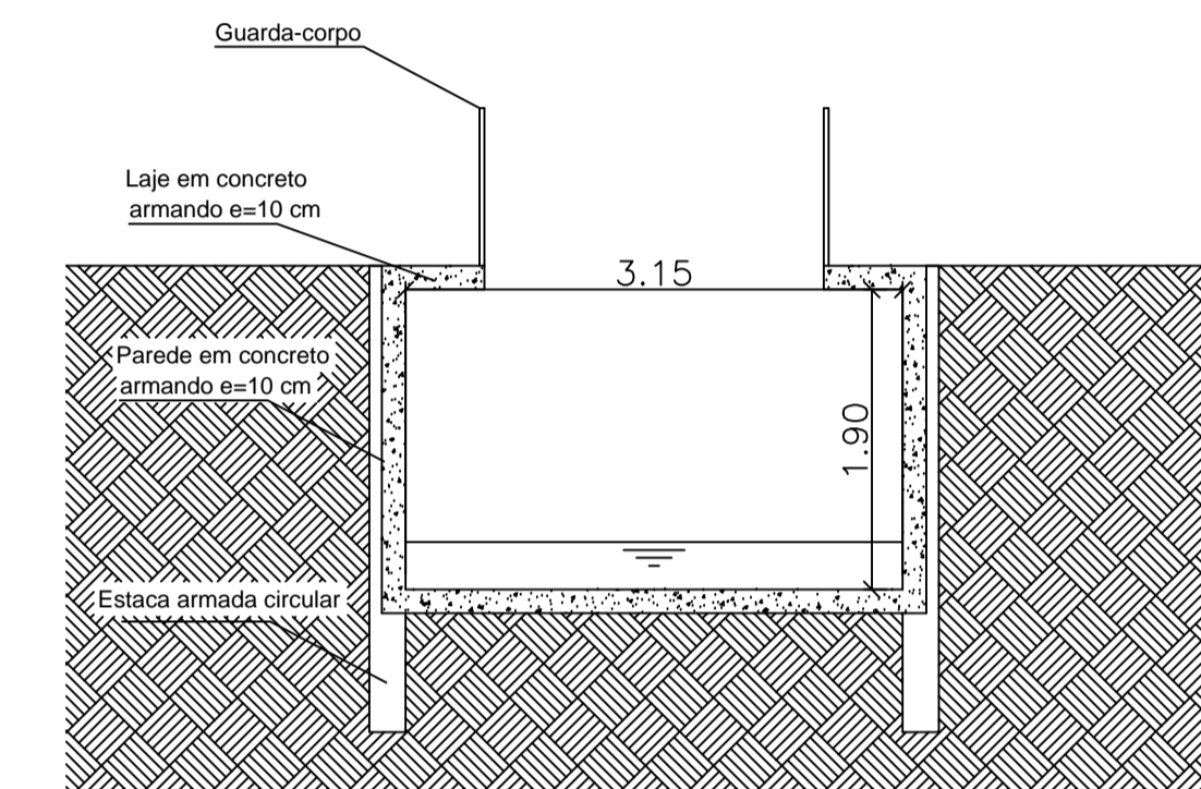
Trecho15 Escala 1: 50
