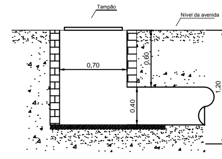
DETALHE POÇO DE VISITA 1 ESC. 1:20
