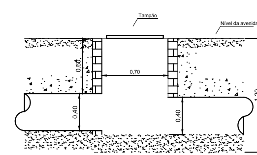
DETALHE POÇO DE VISITA 4 ESC. 1:20
