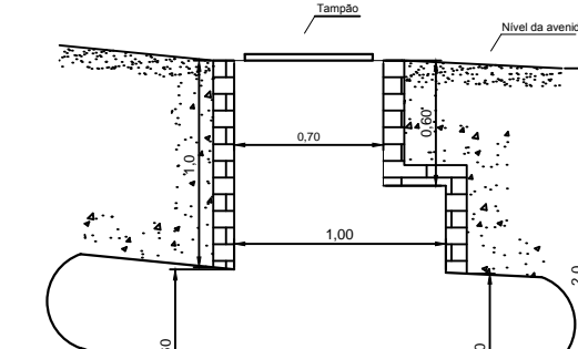
DETALHE POÇO DE VISITA 9 ESC. 1:20
