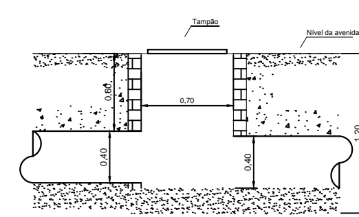
DETALHE POÇO DE VISITA 6 ESC. 1:20
