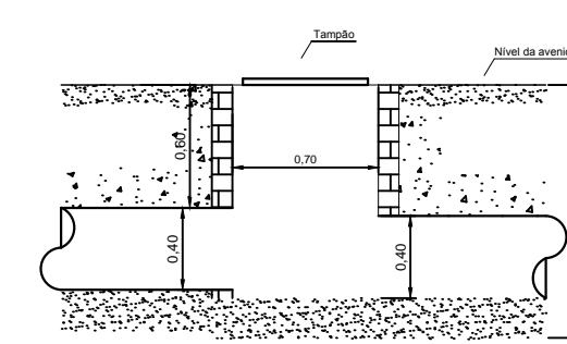
DETALHE POÇO DE VISITA 7 ESC. 1:20
