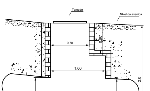
DETALHE POÇO DE VISITA 12 ESC. 1:20
