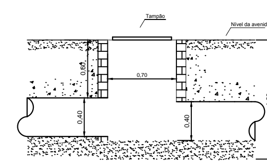
DETALHE POÇO DE VISITA 3 ESC. 1:20
