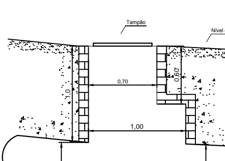
DETALHE POÇO DE VISITA 15 ESC. 1:20
