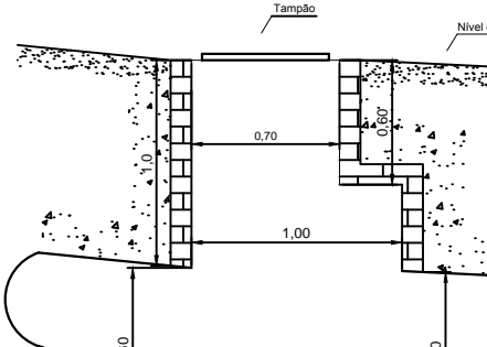
DETALHE POÇO DE VISITA 8 ESC. 1:20
