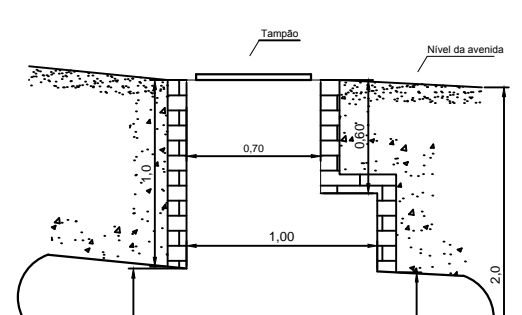
DETALHE POÇO DE VISITA 11 ESC. 1:20
