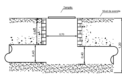
DETALHE POÇO DE VISITA 2 ESC. 1:20
