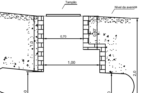
DETALHE POÇO DE VISITA 10 ESC. 1:20
