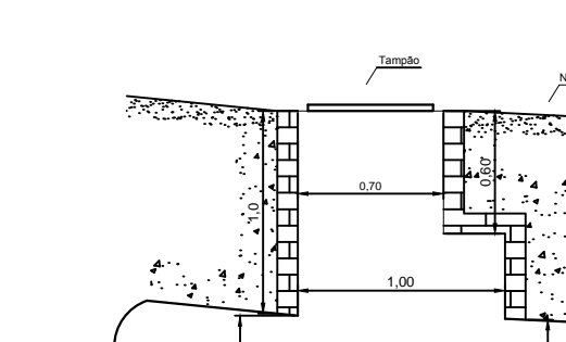
DETALHE POÇO DE VISITA 14 ESC. 1:20
