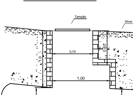
DETALHE POÇO DE VISITA 13 ESC. 1:20
