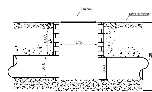
DETALHE POÇO DE VISITA 5 ESC. 1:20
