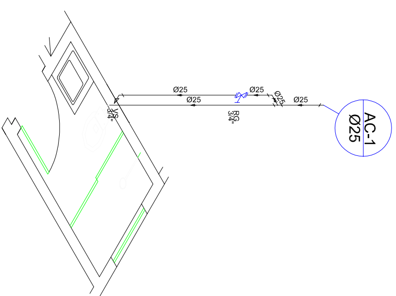
Detalhe H1=H2 Escala 1:50
