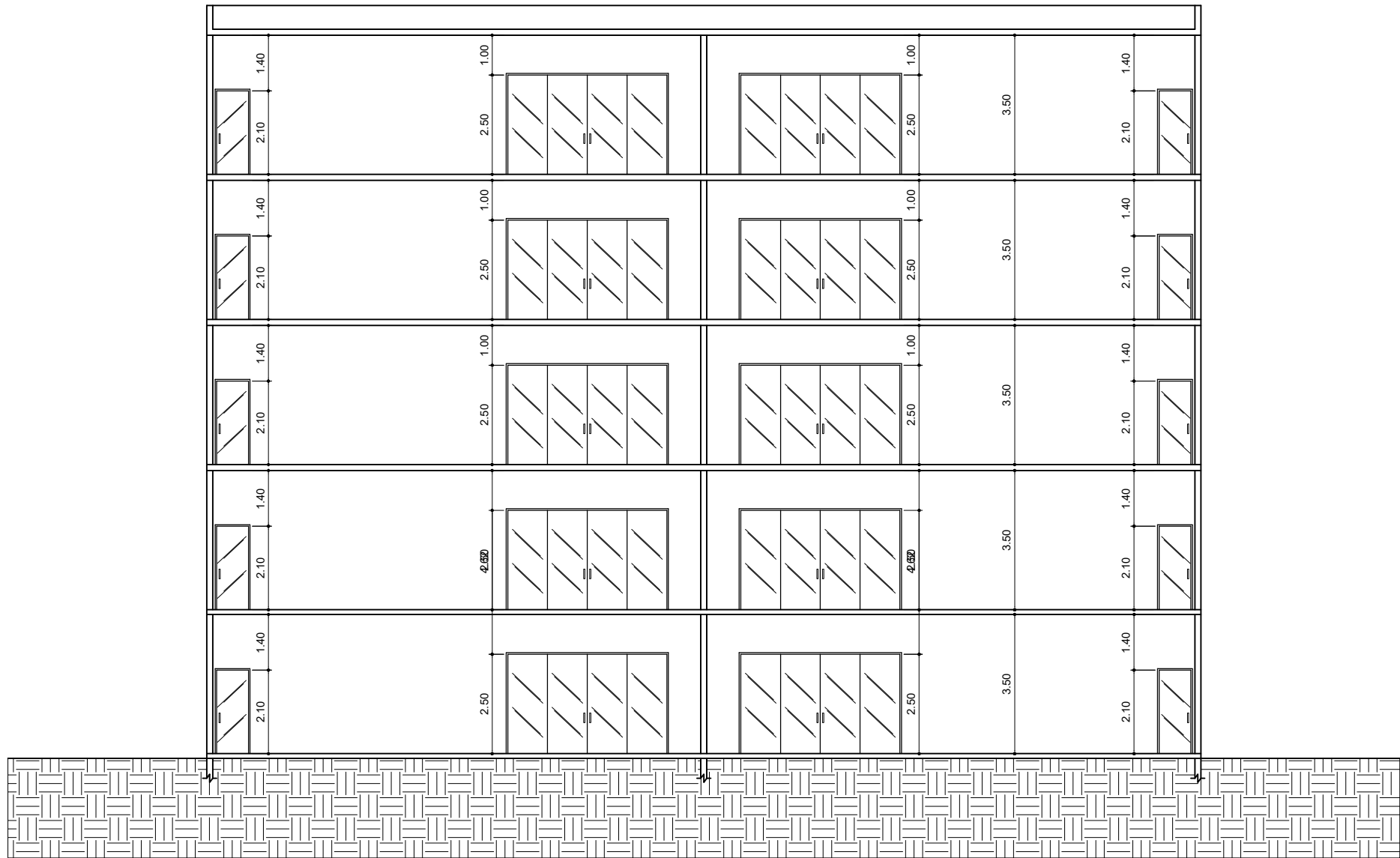
FIGURA 02 - CORTE AB ESCALA 1/100
