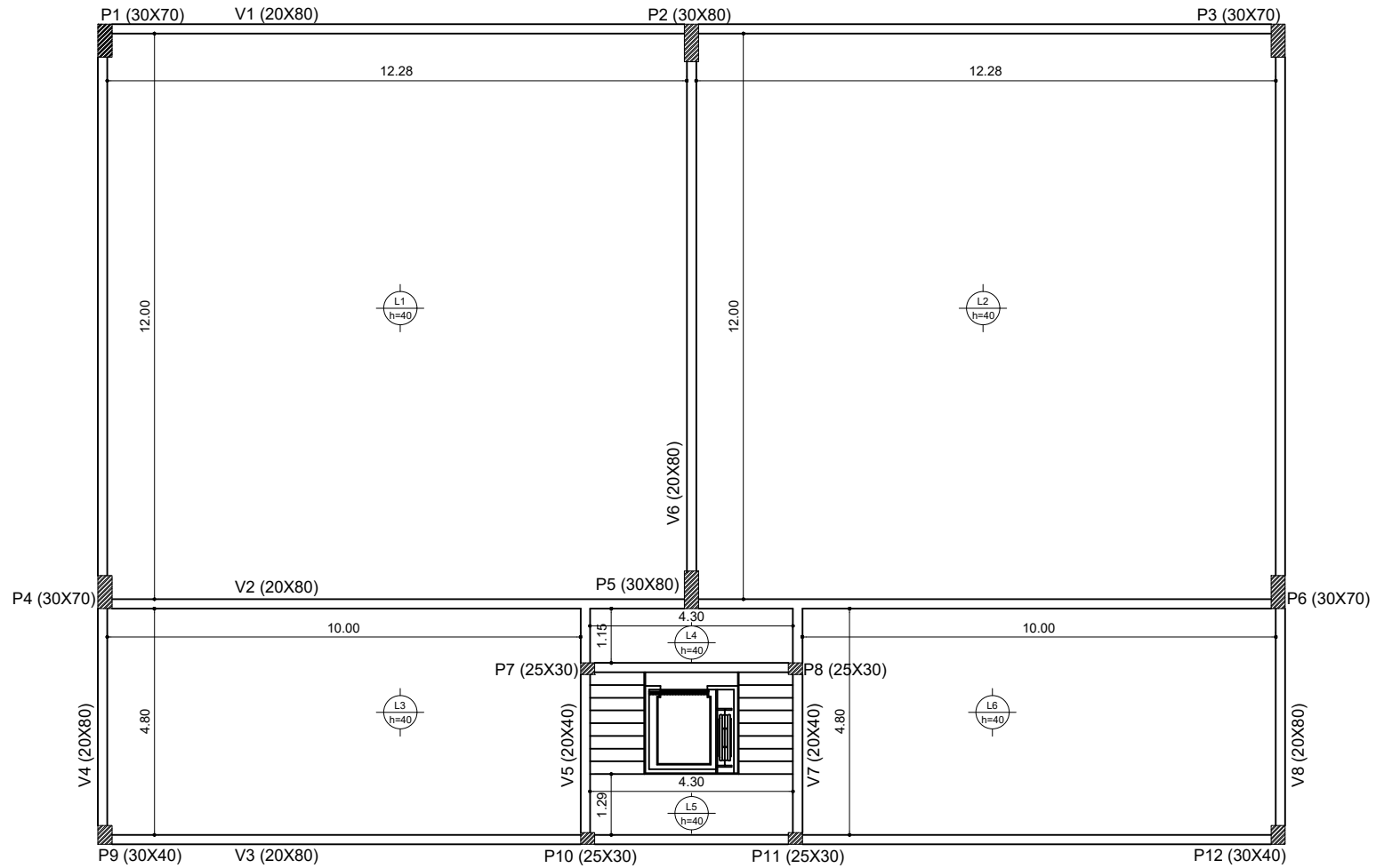
FIGURA 01 - PLANTA DE FORMA - LAJE ALVEOLAR ESCALA 1/100
